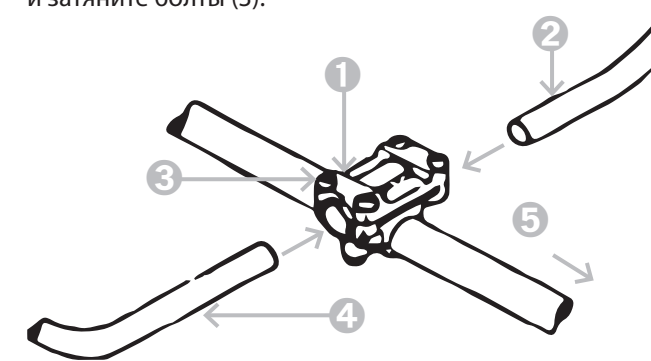
Рисунок 4.1. Установка U-образной рукоятки
