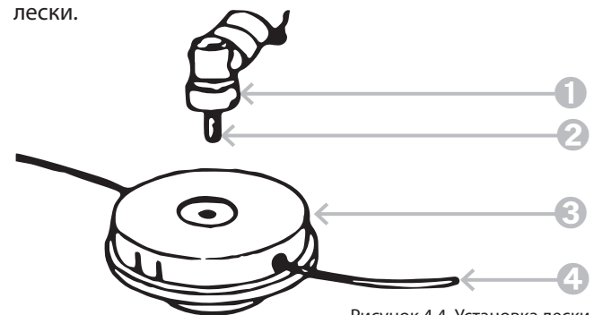
Рисунок 4.4. Установка лески
