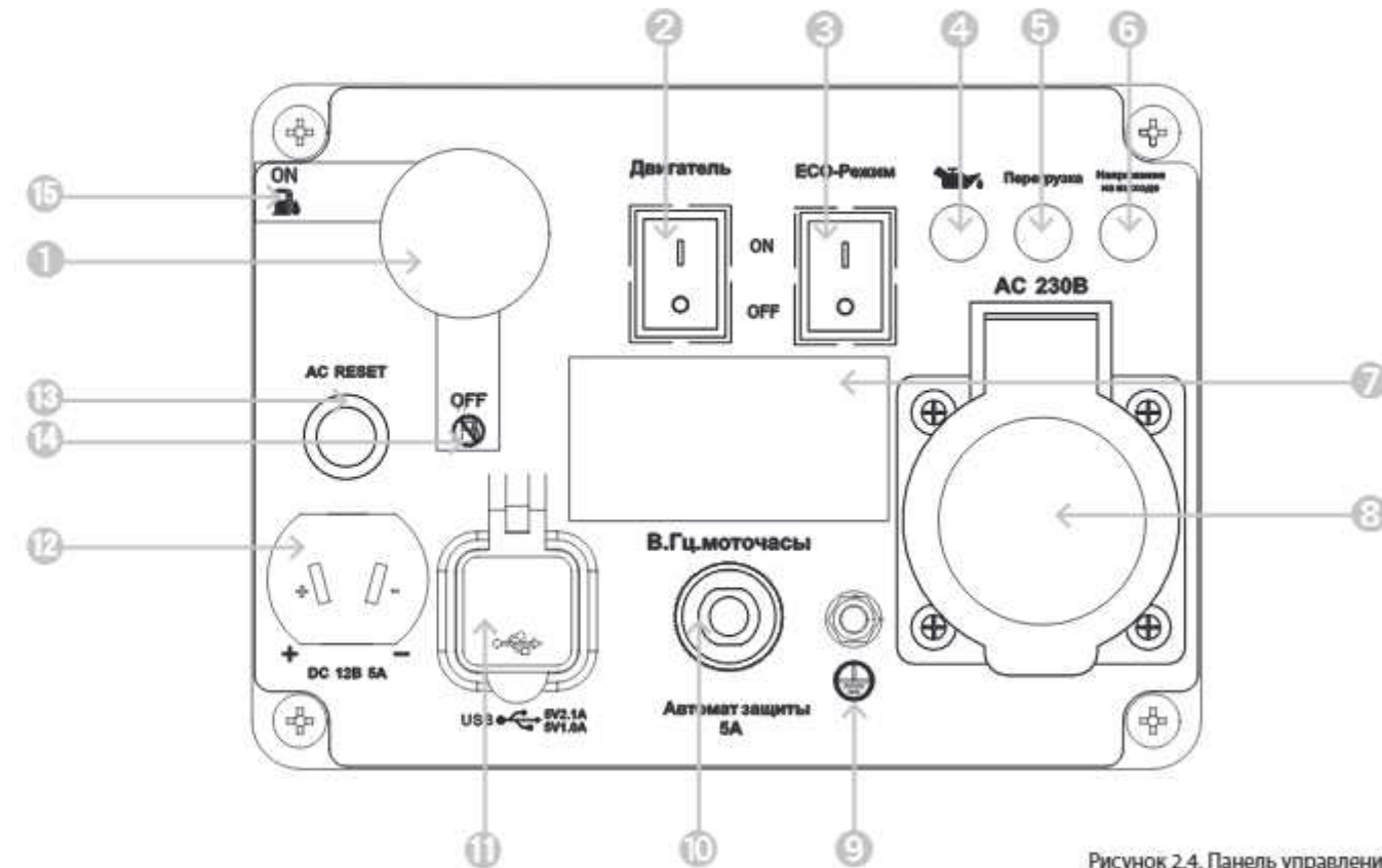
Рисунок 2.4. Панель управления
